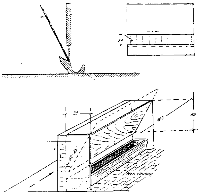
Sơ đồ kiểu máng ăn bán tự động
